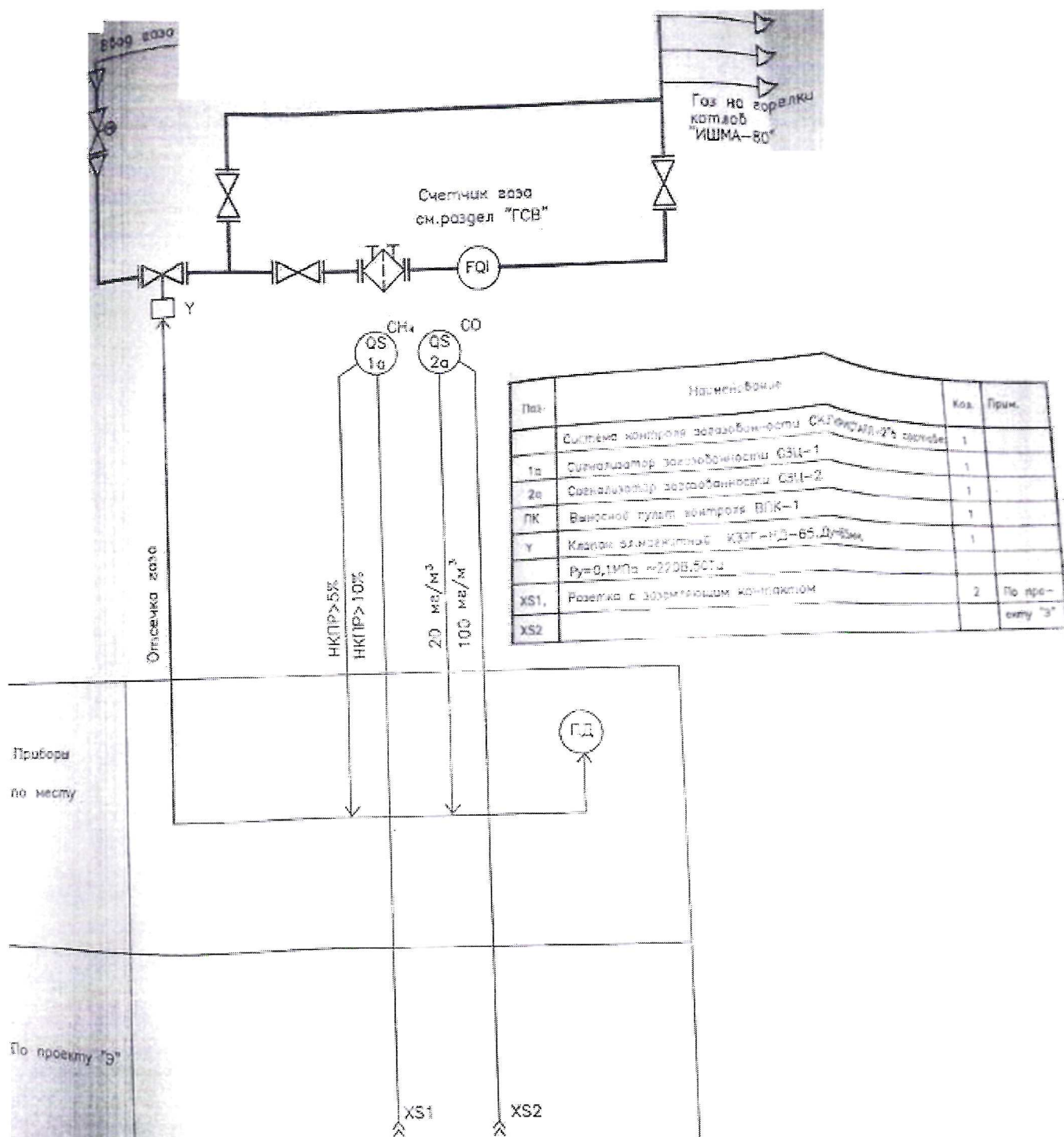
Рисунок 4 - Схема приборов контроля загазованности котельной.
